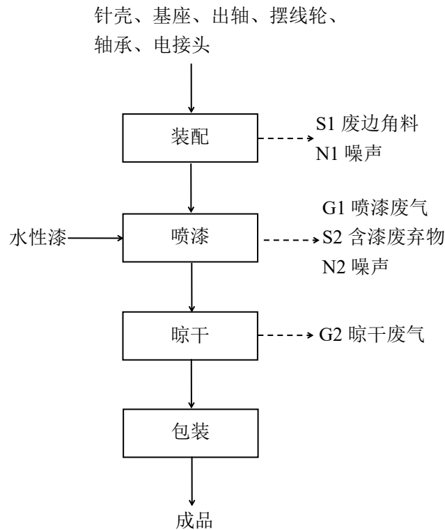
图 2-2 减速机生产工艺流程图
